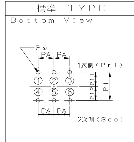
ピン仕様図 (Bottom View)
