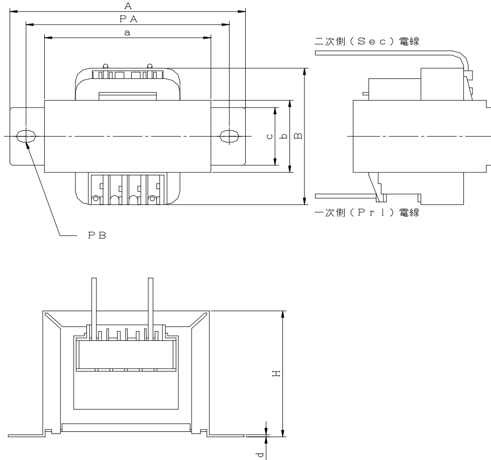
参考外形図 FCT35-TYPE
